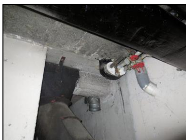
Photo N° 940 AMIANTE CIMENT -- LOCAL VO -1 Gaines & coffres horizontaux Coude de ventilation haute (Fibres-ciment)
